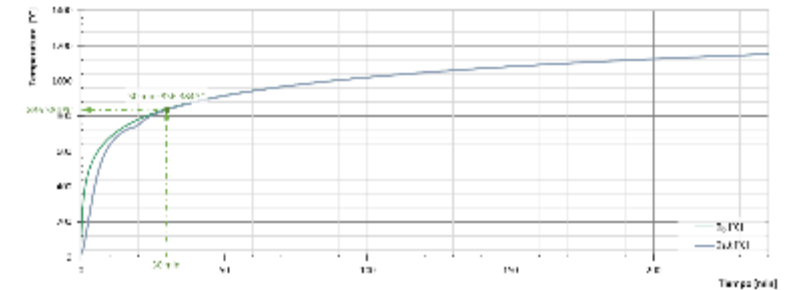
Evolución de temperaturas en perfil
