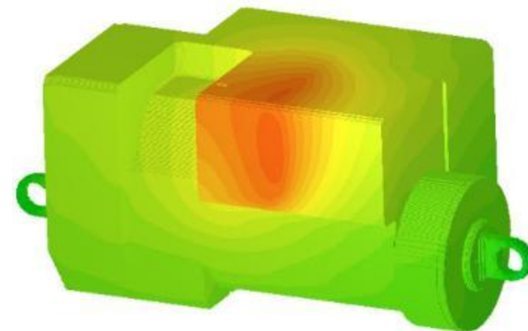
Temperatura superficial en carcasa
