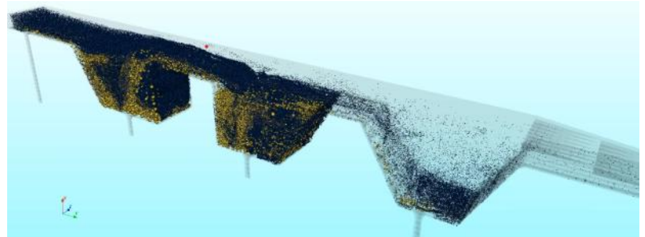
Simulación del proceso de captación de partículas suspendidas
