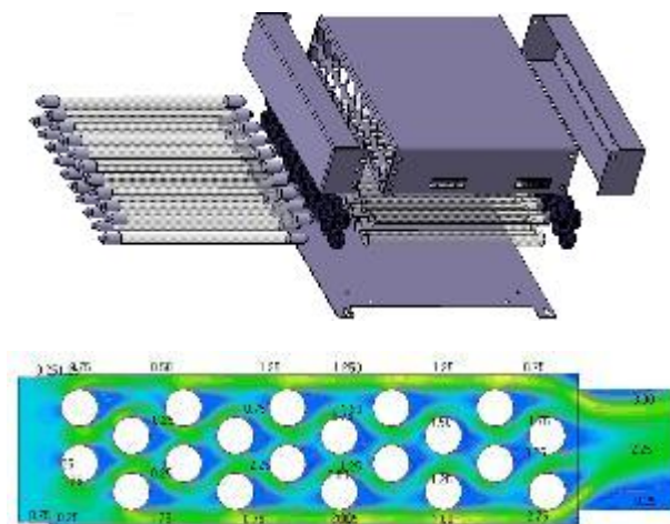
Simulación CFD
