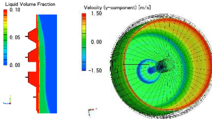
Superficie libre del fluido en rotación
