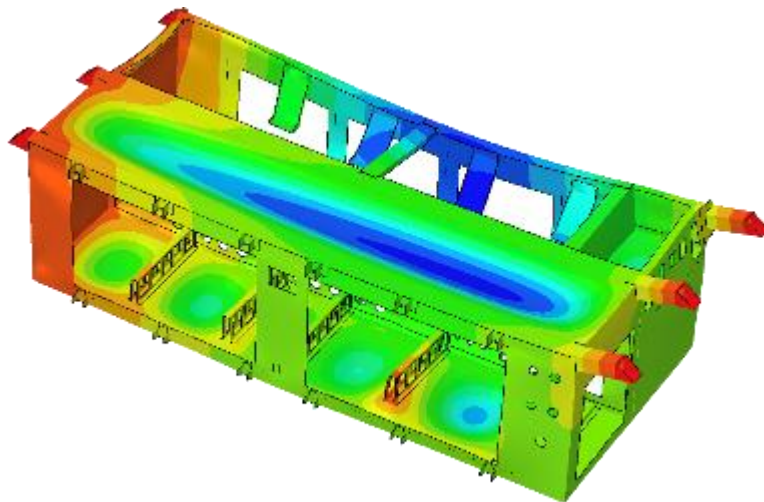
3D y Campo de Deformaciones
