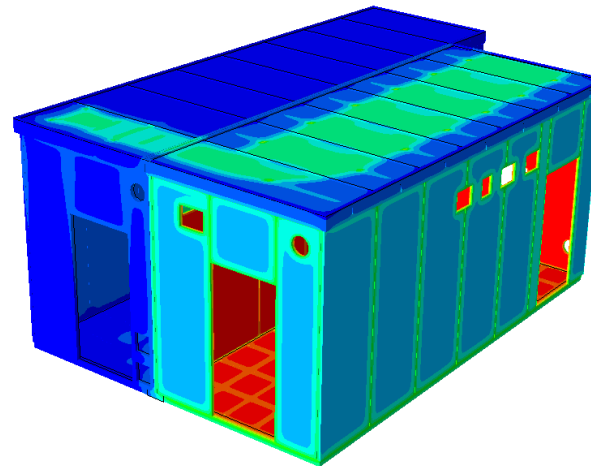
Campo de temperaturas – Carga fuego t=1800s
