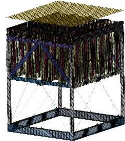
Modelo FEM
