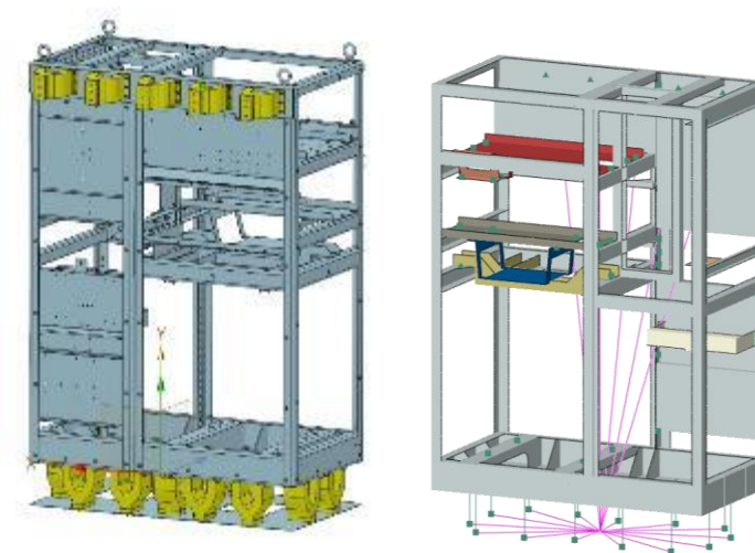
CAD y FEM
