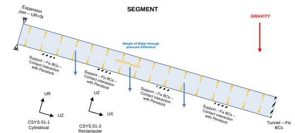
Esquema de cargas
