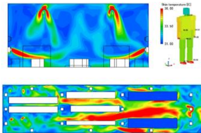
Mapas de velocidad y temperatura
