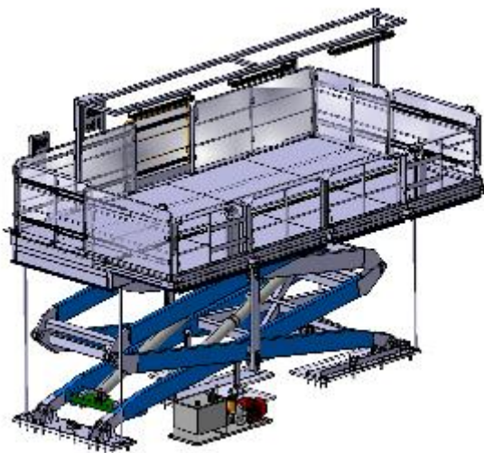
Diseño 3D
