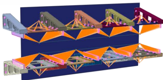
Modelos FEM
