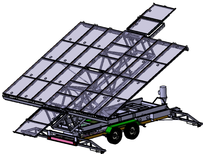
Diseño 3D
