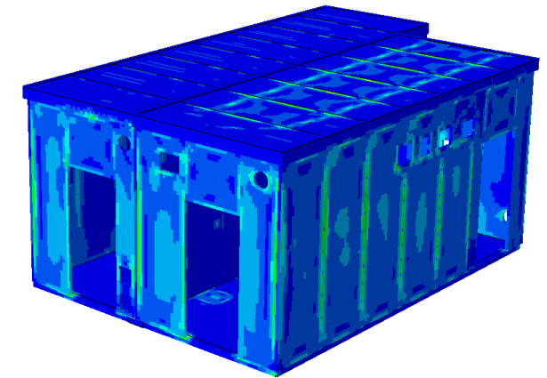
Campo de tensiones Von Mises
