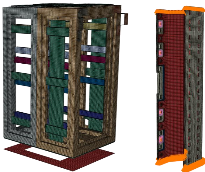
Modelo FEM
