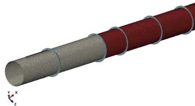
Modelo FEM
