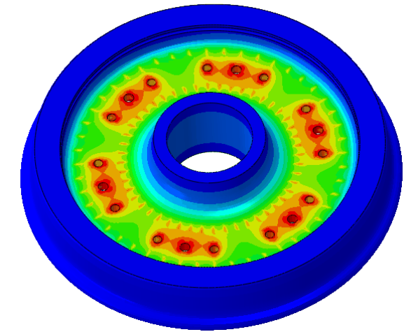
Frenada de emergencia. Temperaturas
