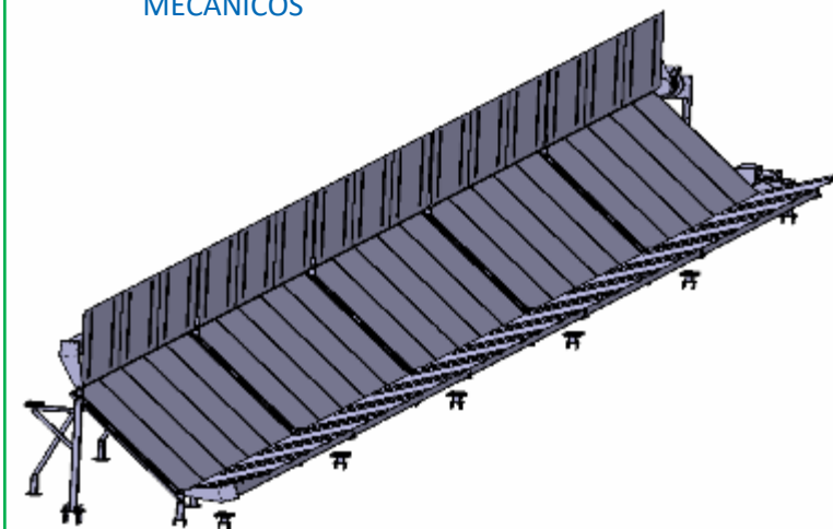
Diseño Colector 5m
