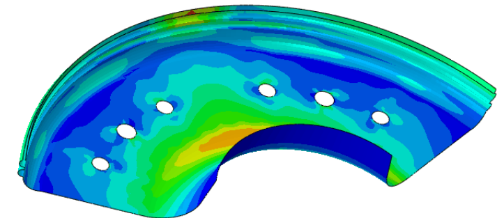
Fatiga uniaxial – Rango de tensiones
