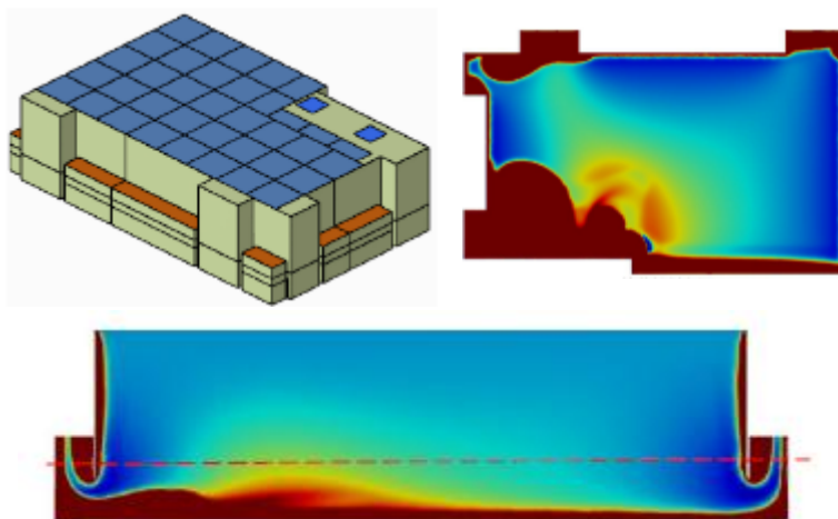
Mapas de flujo en la sala estudiada
