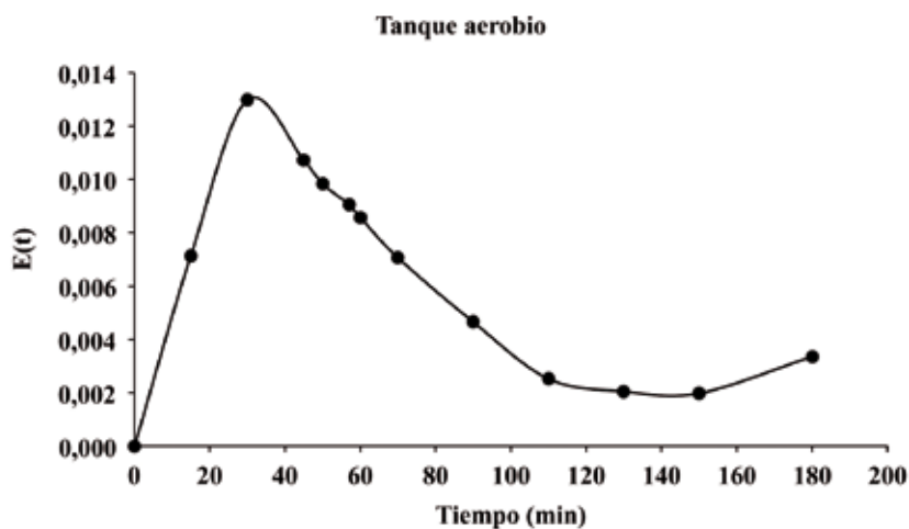
FIGURA 3. Distribución del tiempo de residencia de las partículas de trazador a la salida del tanque aerobio.
