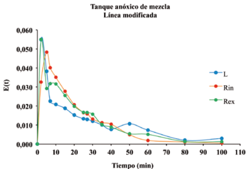
FIGURA 8. Distribuciones del tiempo de residencia del trazador a la salida del tanque anóxico de mezcla con la recirculación interna superficial.
