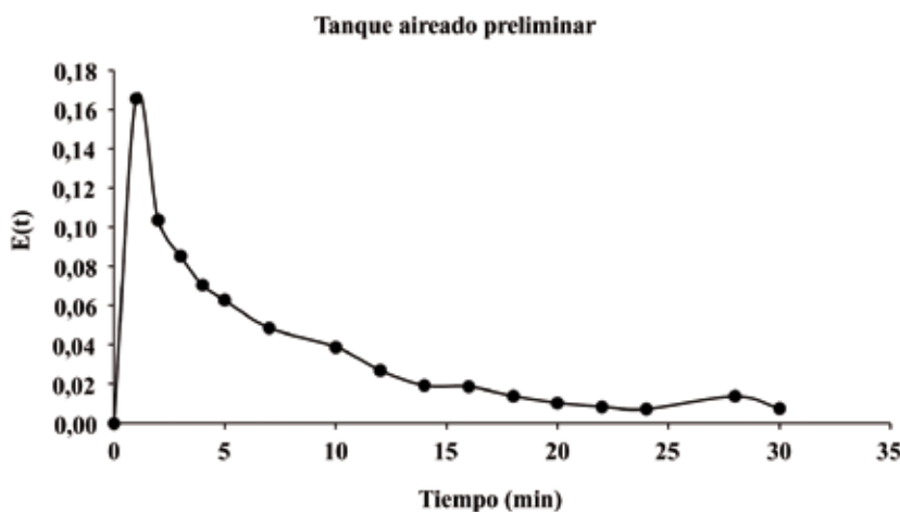
FIGURA 4. Distribución del tiempo de residencia del trazador en el tanque aireado preliminar.
