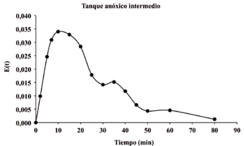
FIGURA 6. Distribución del tiempo de residencia del trazador en el tanque anóxico intermedio.
