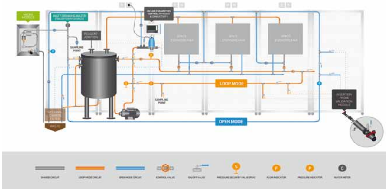
FIGURA 3. Diagrama del circuito hidráulico de la Plataforma de Validación de Sensores. Fuente: Cetaqua.
