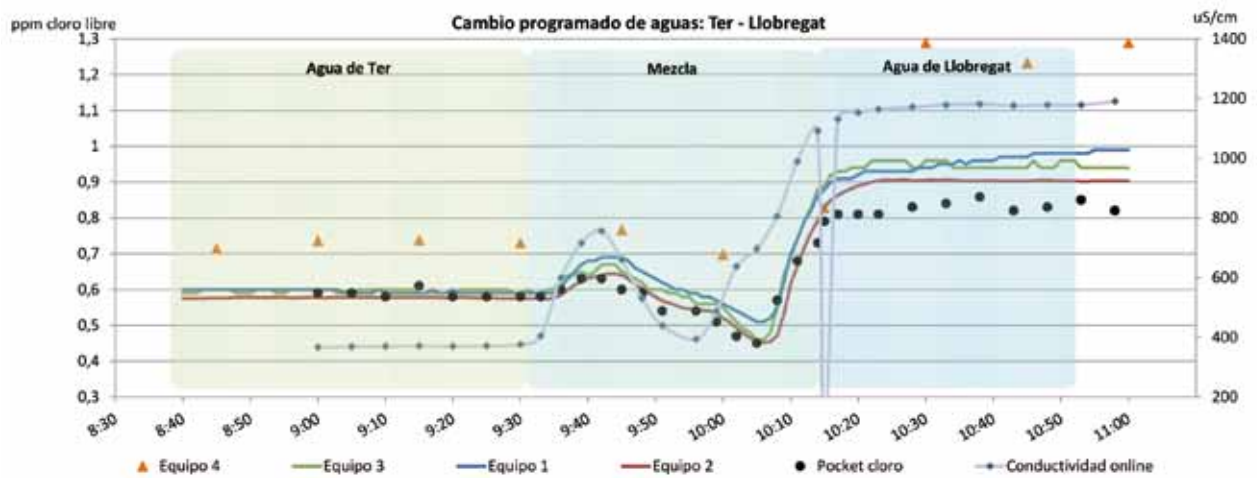
FIGURA 10. Prueba de validación de los sensores de cloro: cambio de matriz de aguas. Fuente: Cetaqua.
