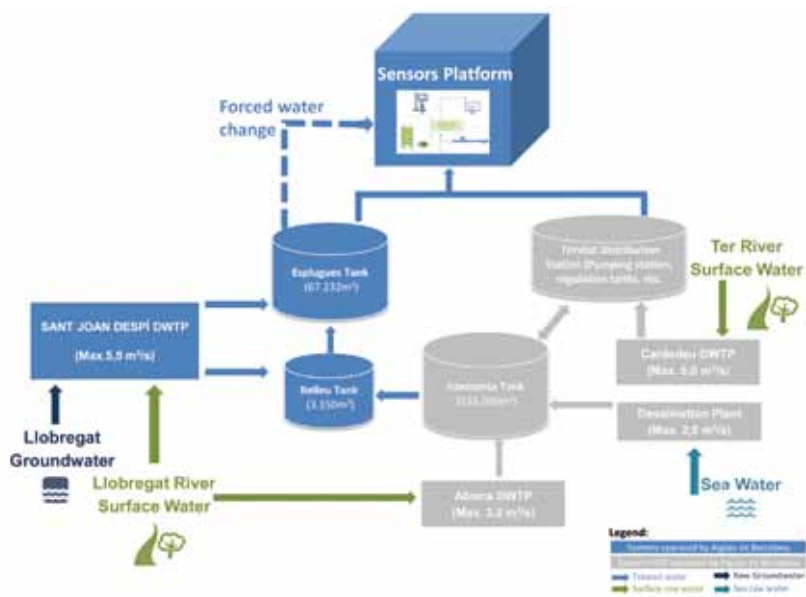
FIGURA 2. Diagrama hidráulico de la alimentación de la plataforma de sensores. Fuente: Cetaqua.
